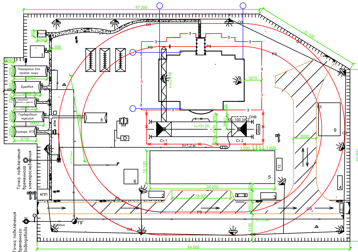
Экспликация временных зданий и сооружений
