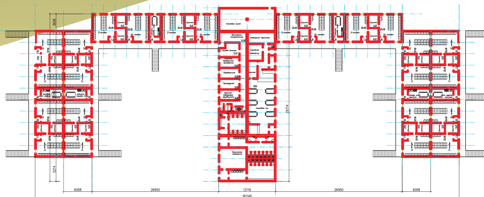
БЫТОВОЙ КОРПУС С САНИТАРНО- -БЫТОВЫМИ ПОМЕЩЕНИЯМИ
