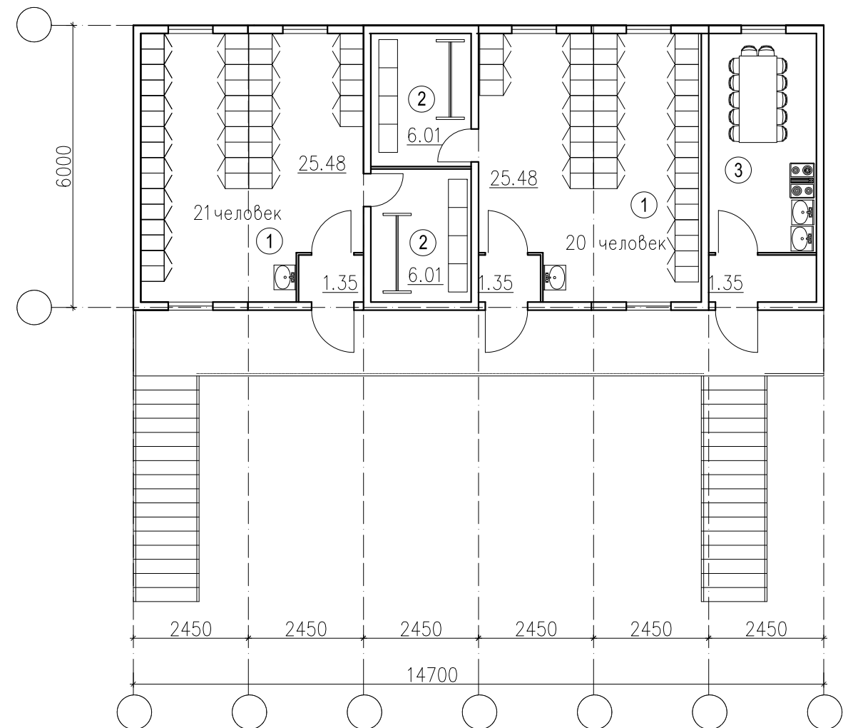
План верхнего уровня
