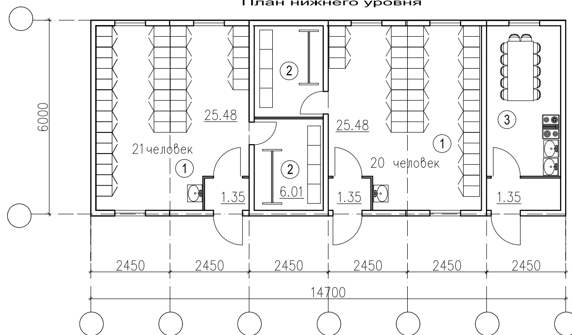
План нижнего уровня
